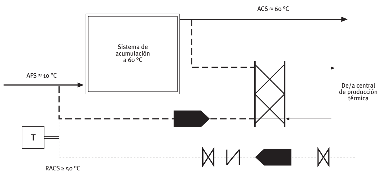
Fig. 12: Esquema simplificado de preparación de ACS a 60\text{ }^{\circ}\text{C}
